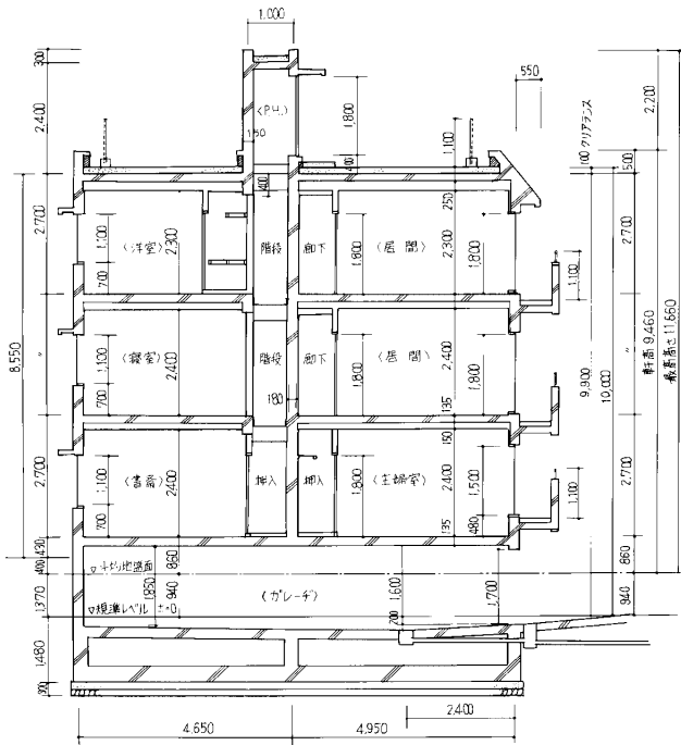
断面図(1)
