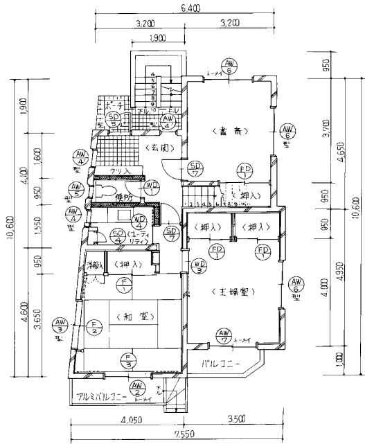
1階平面図
