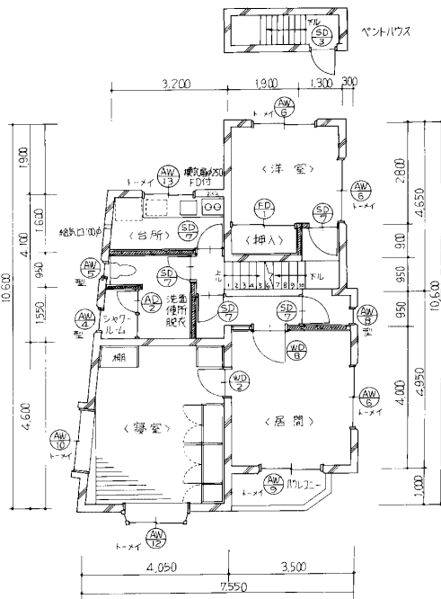
3階平面図
