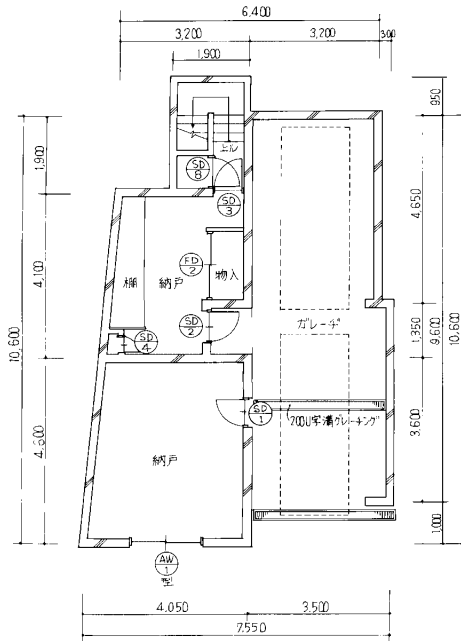
地階平面図
