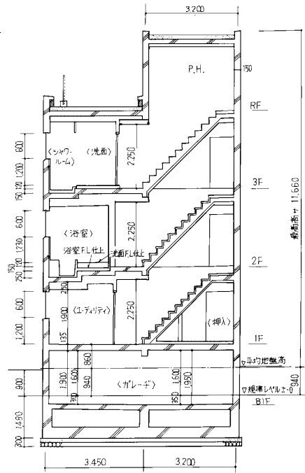
断面図(2)
