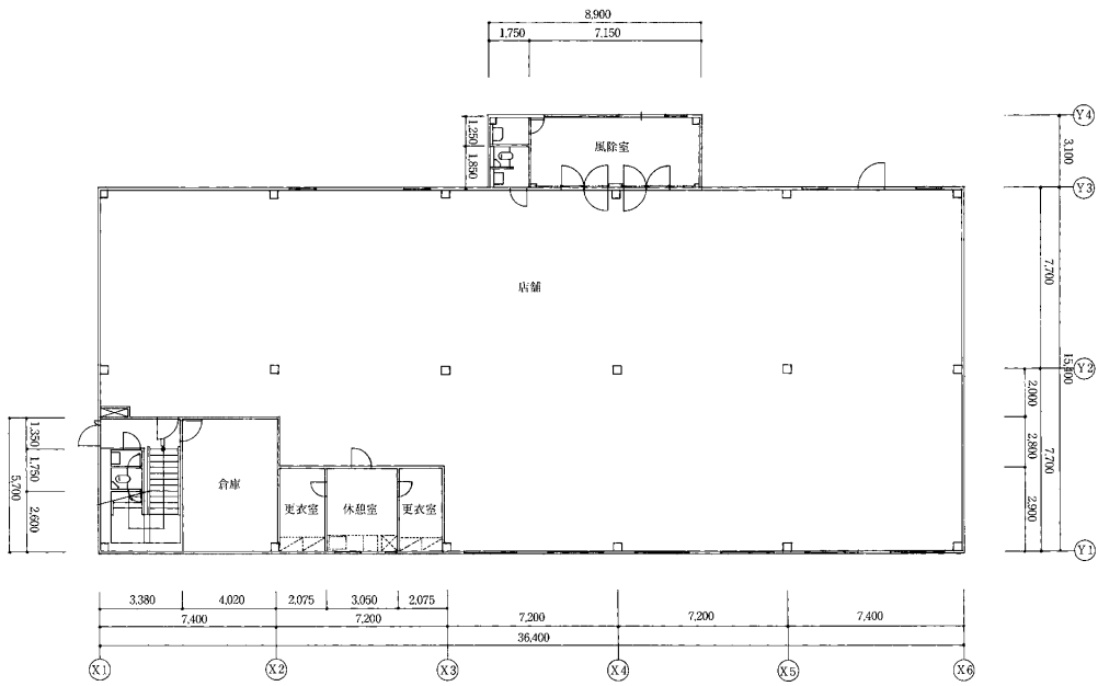
2 階平面図
