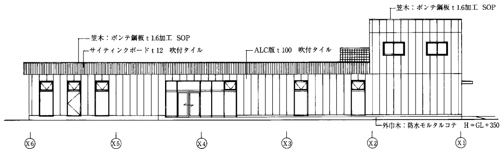
南立面図
