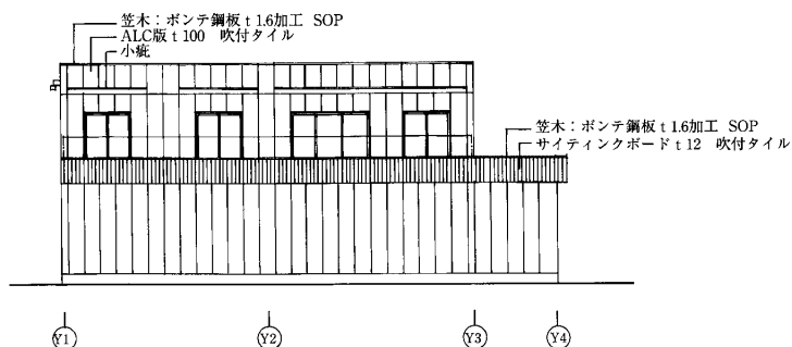
西立面図
