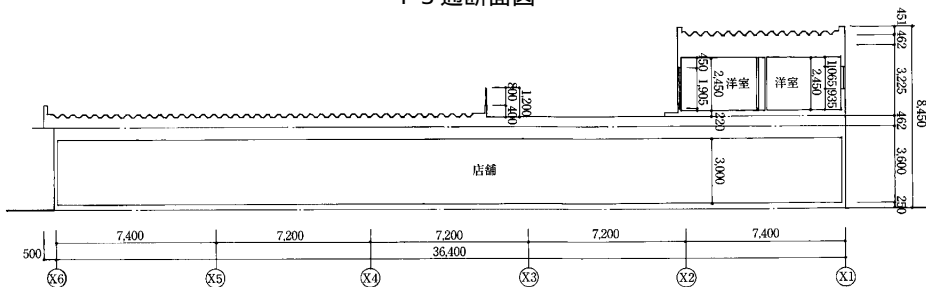
Y 3 通断面図
